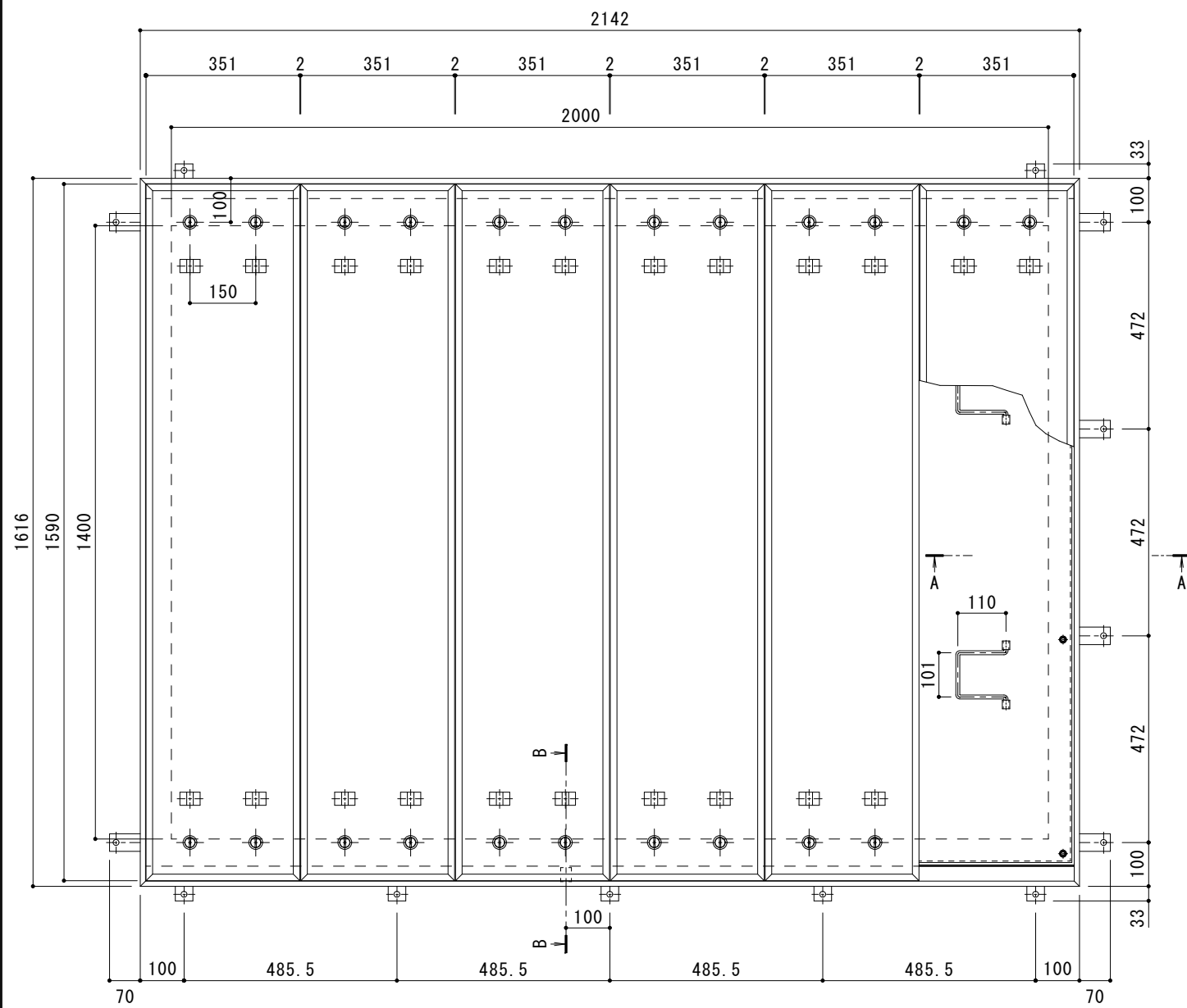
平面詳細図 S = 1 : 10
