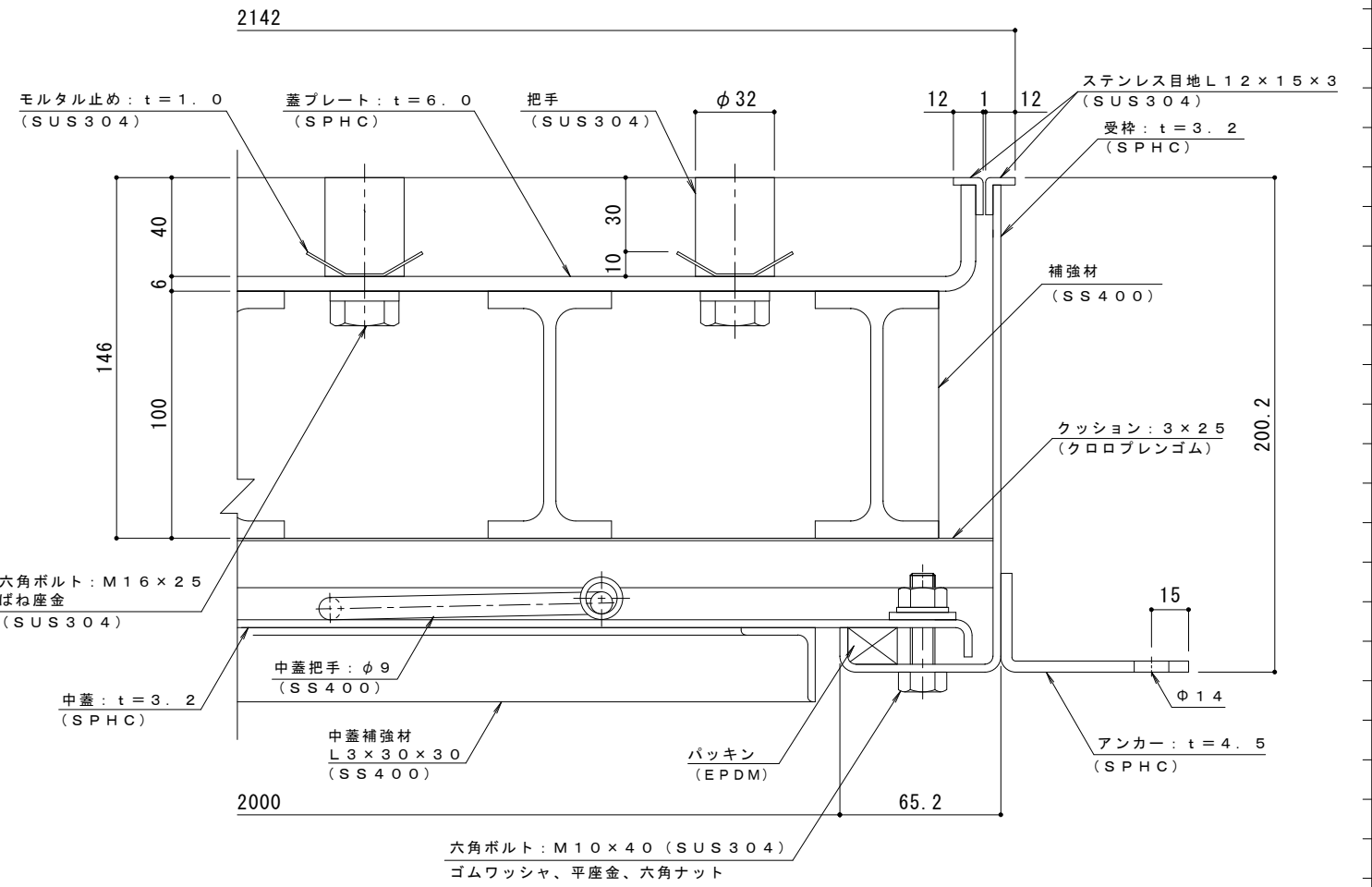
A-A断面詳細図 S = 1 : 2
