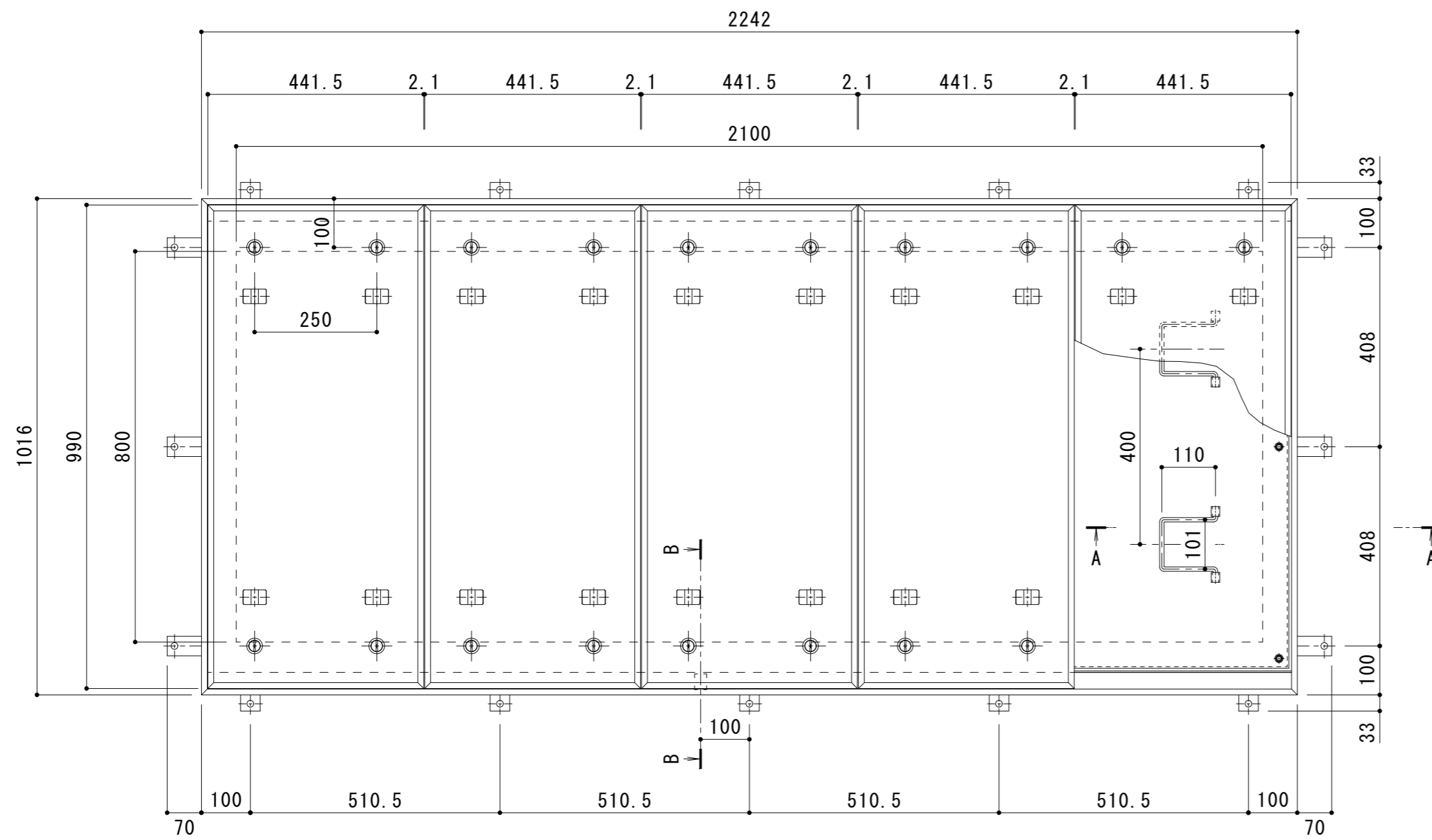
平面詳細図 S = 1 : 1 0
