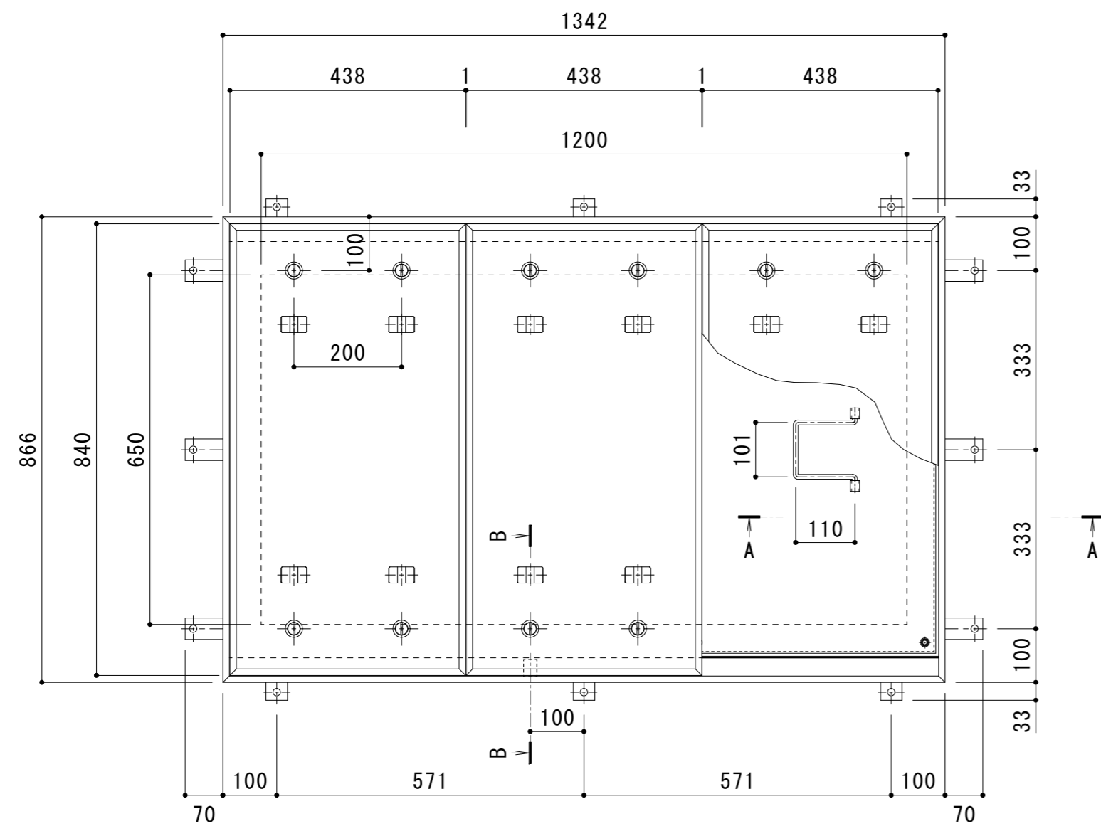
平面詳細図 S = 1 : 10
