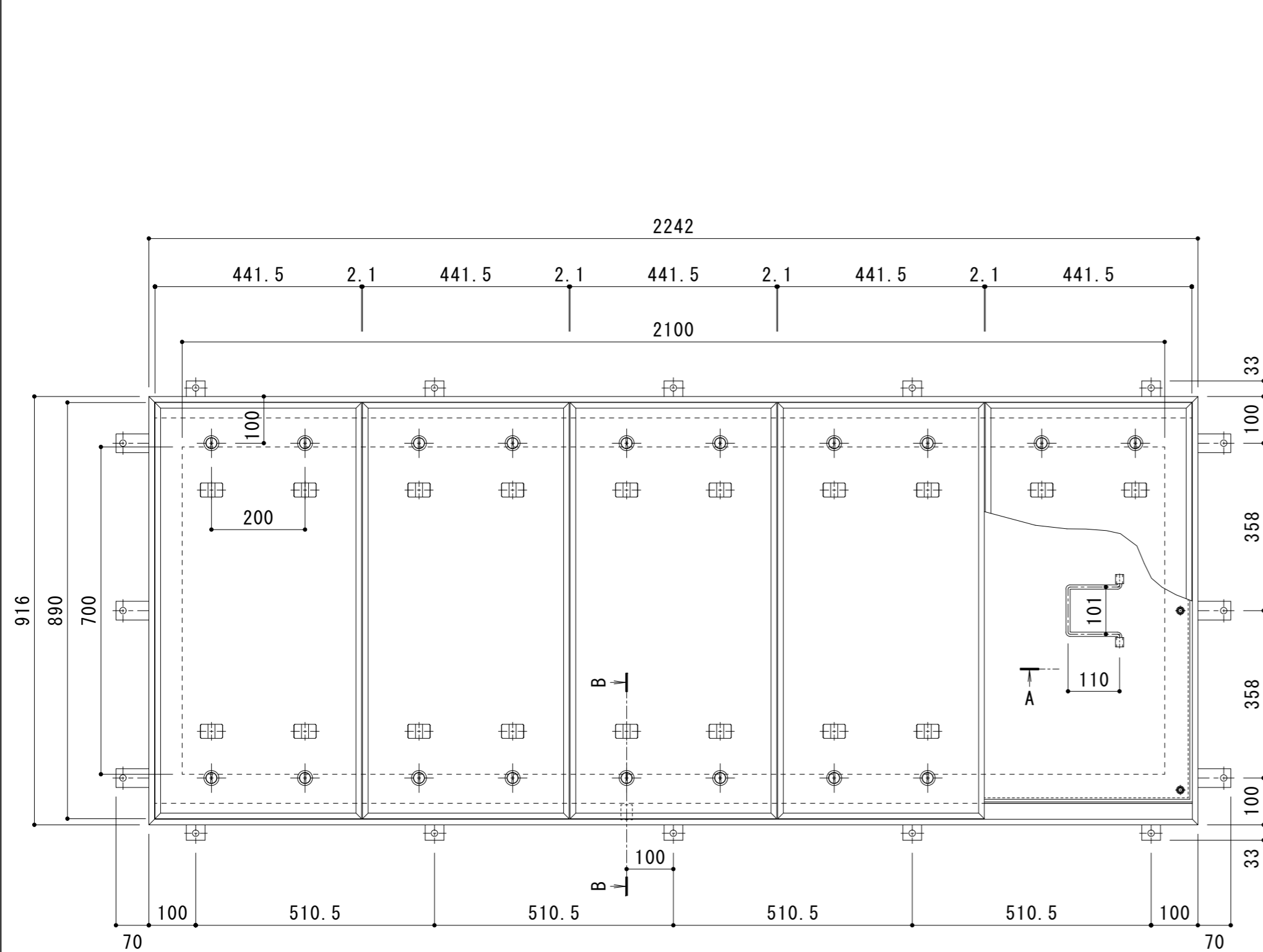
平面詳細図 S = 1 : 1.0
