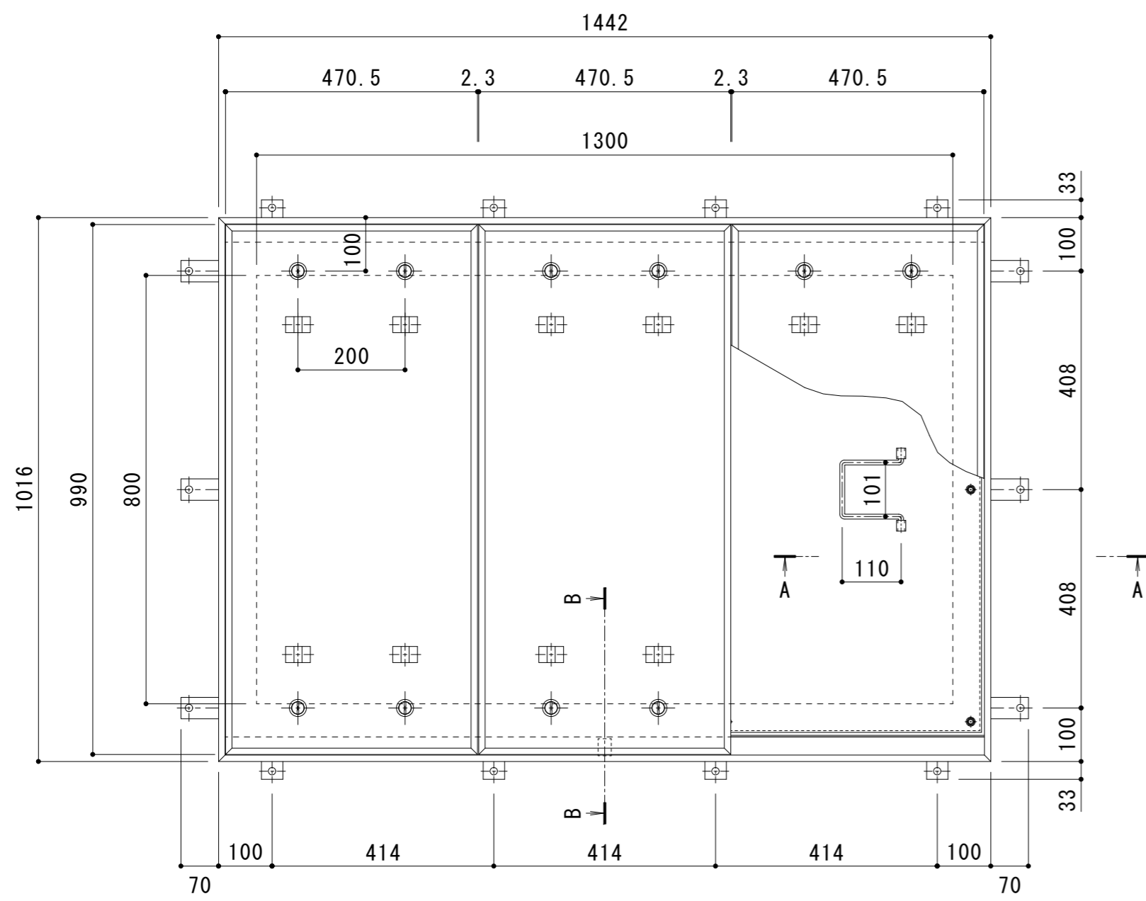
平面詳細図 S = 1 : 10
