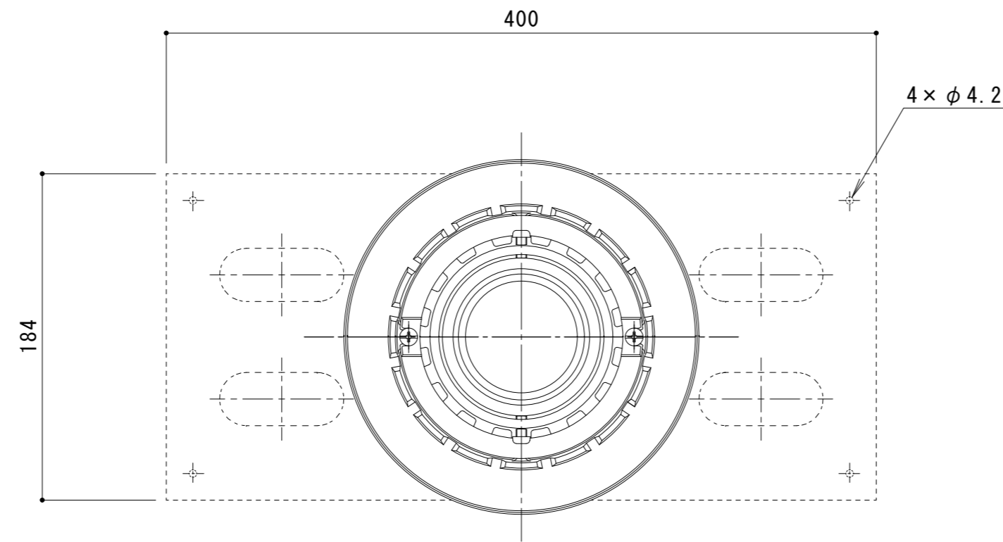
平面図 S = 1 : 3
