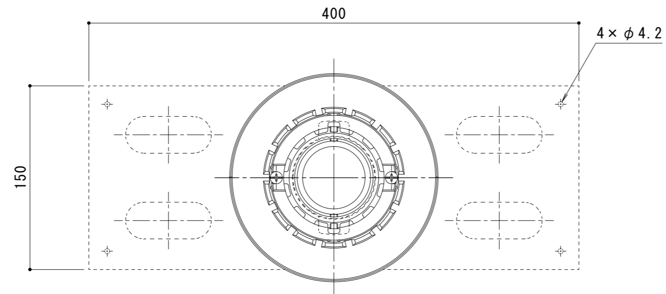
平面図 S = 1 : 3
