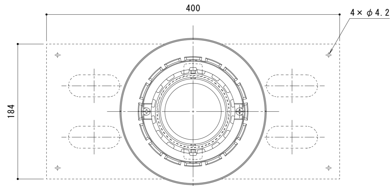
平面図 S = 1 : 3
