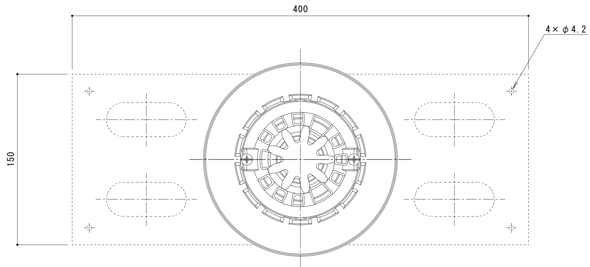
平面図 S = 1 : 2
