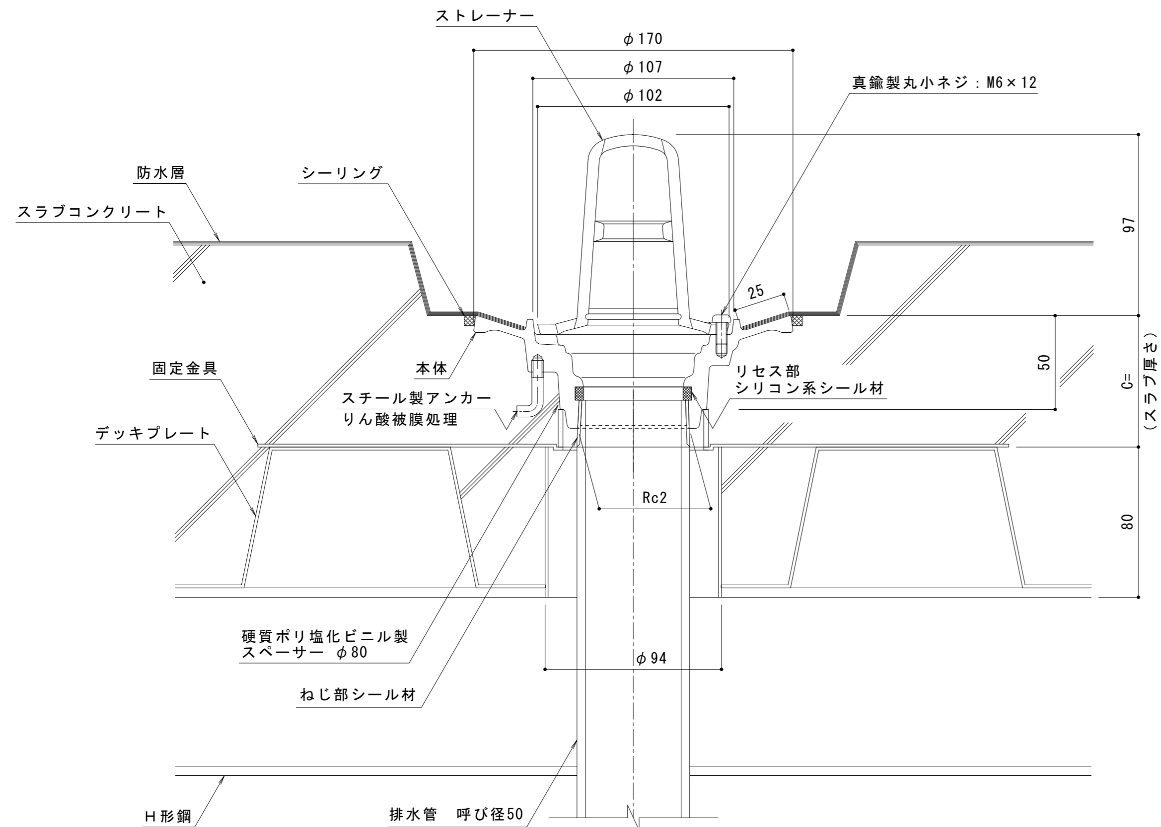
断面図 (納まり) S = 1 : 2
