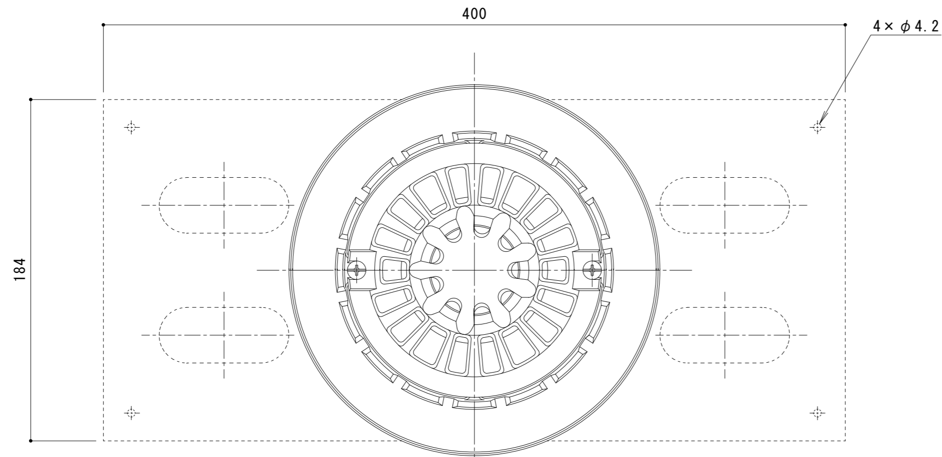
平面図 S = 1 : 2
