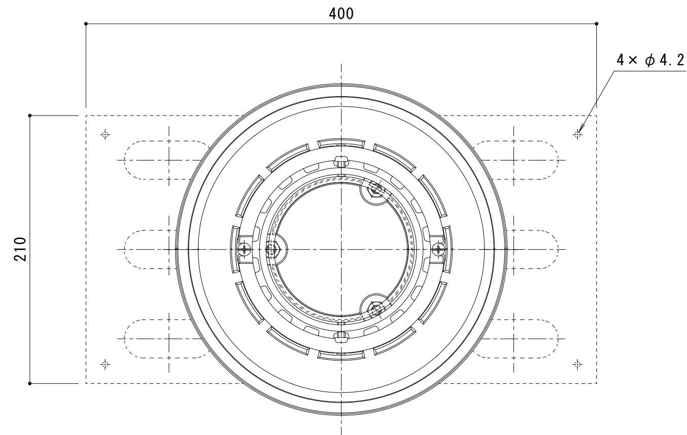
平面図 S = 1 : 3
