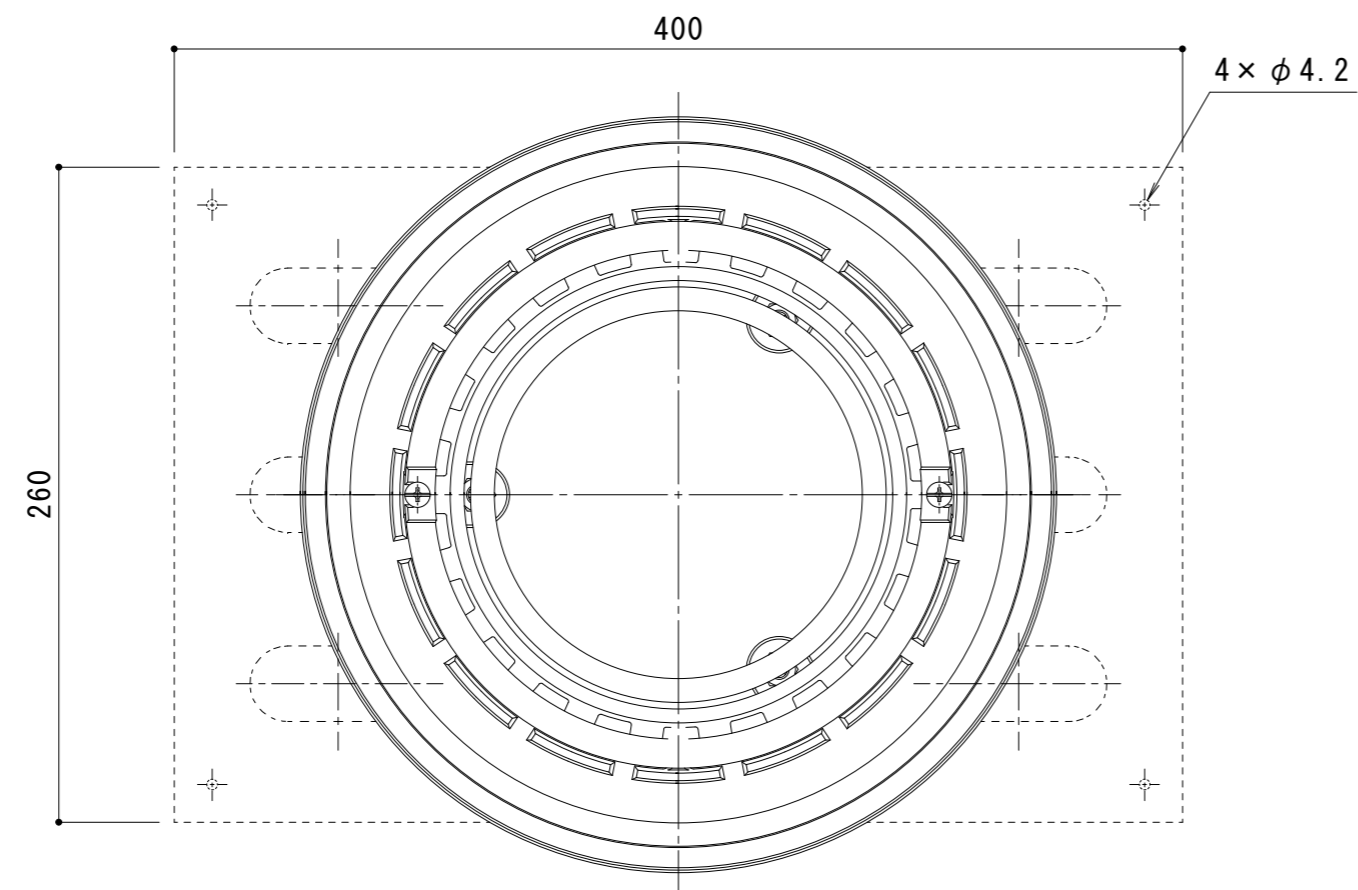
平面図 S = 1 : 3
