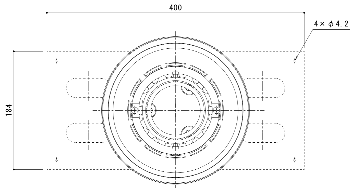
平面図 S = 1 : 3
