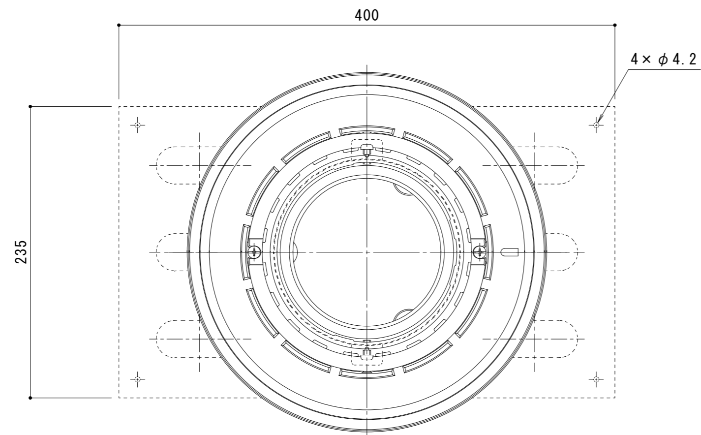
平面図 S = 1 : 3
