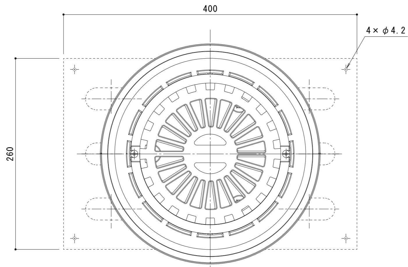
平面図 S = 1 : 3
