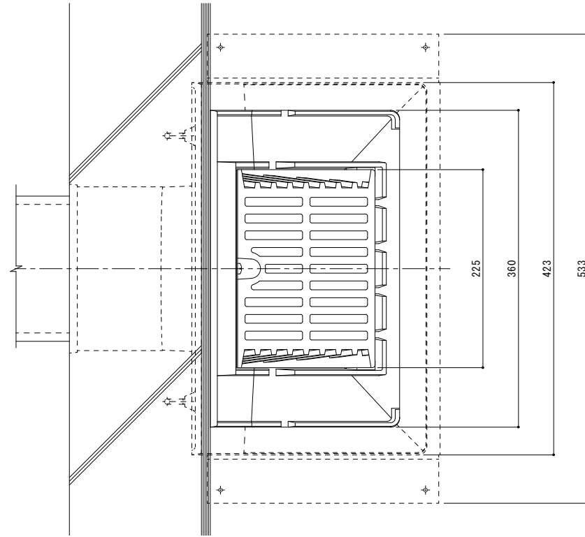
平面図 S = 1 : 3
