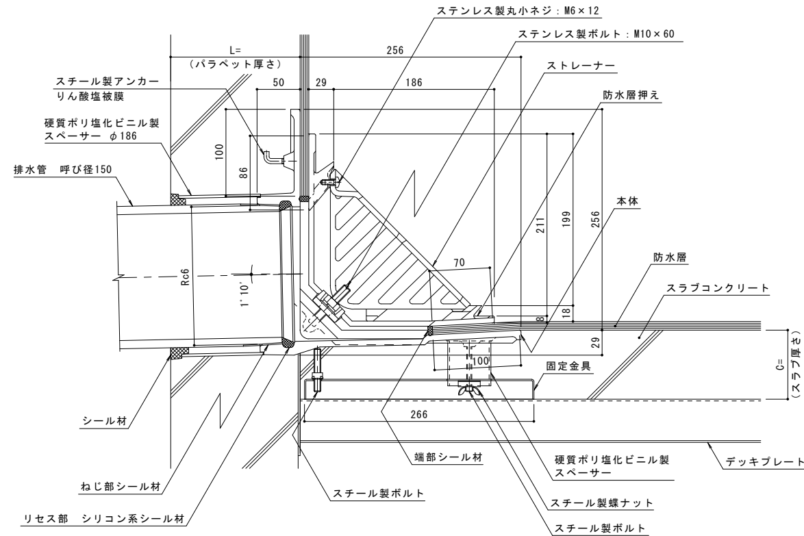
断面図 (納まり) S = 1 : 3
