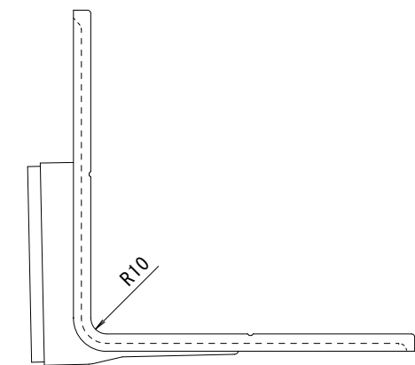
本体コーナー部寸法 S = 1 : 3
