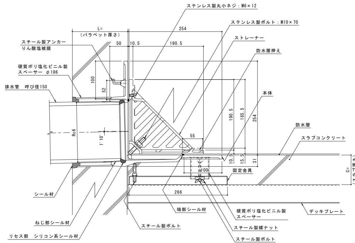
断面図 (納まり) S = 1 : 3
