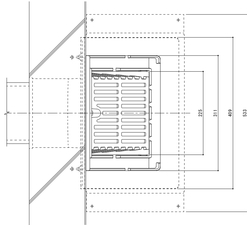
平面図 S = 1 : 3
