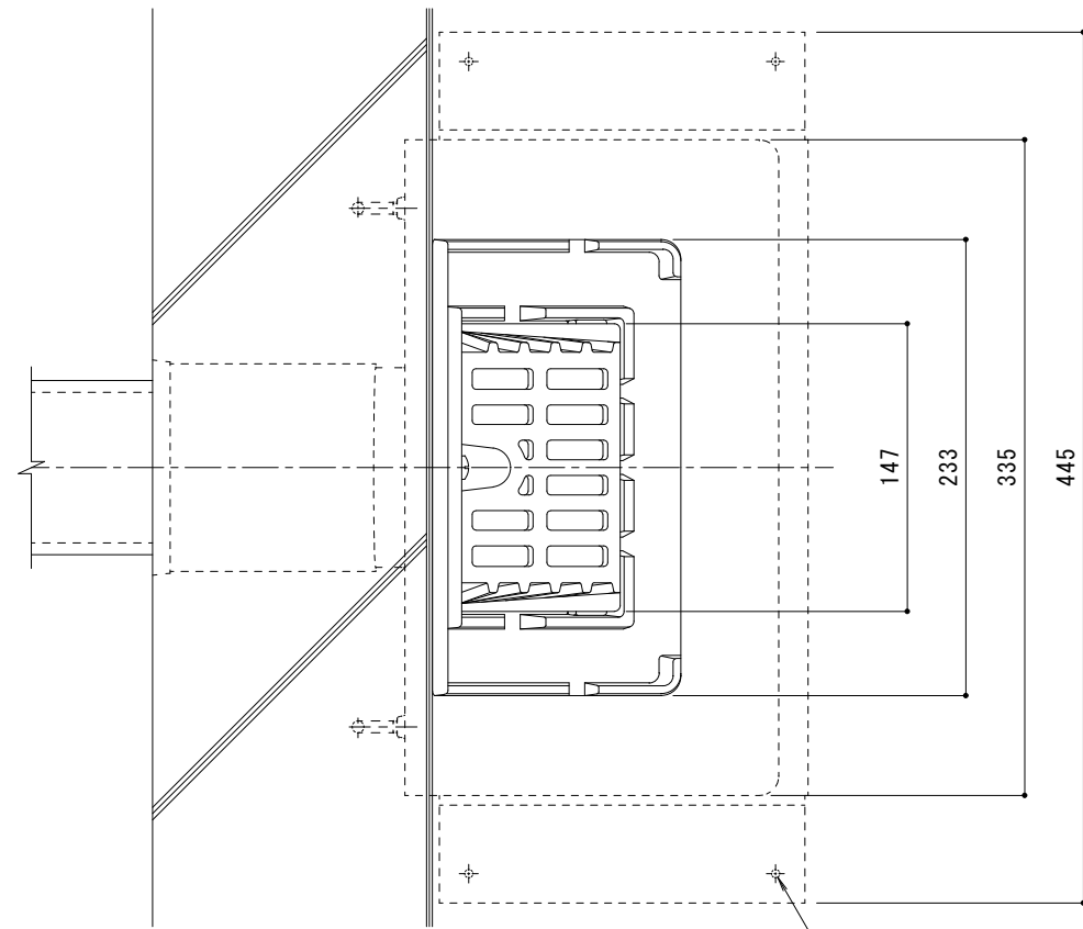
平面図 S = 1 : 3
