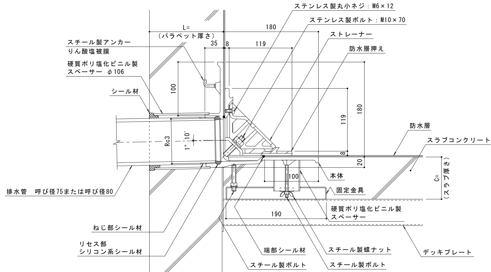
断面図 (納まり) S = 1 : 3
