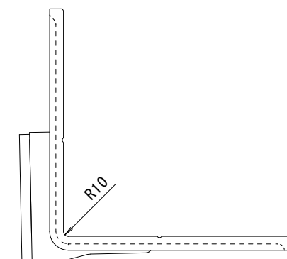
本体コーナー部寸法 S = 1 : 3
