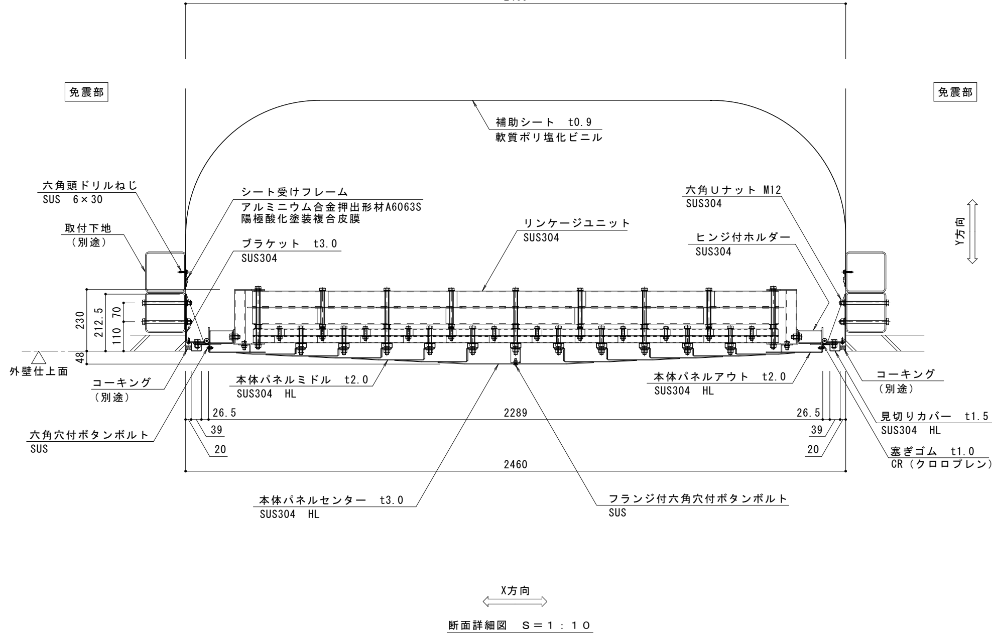
壁部（外壁）製品施工クリアランス 2460
