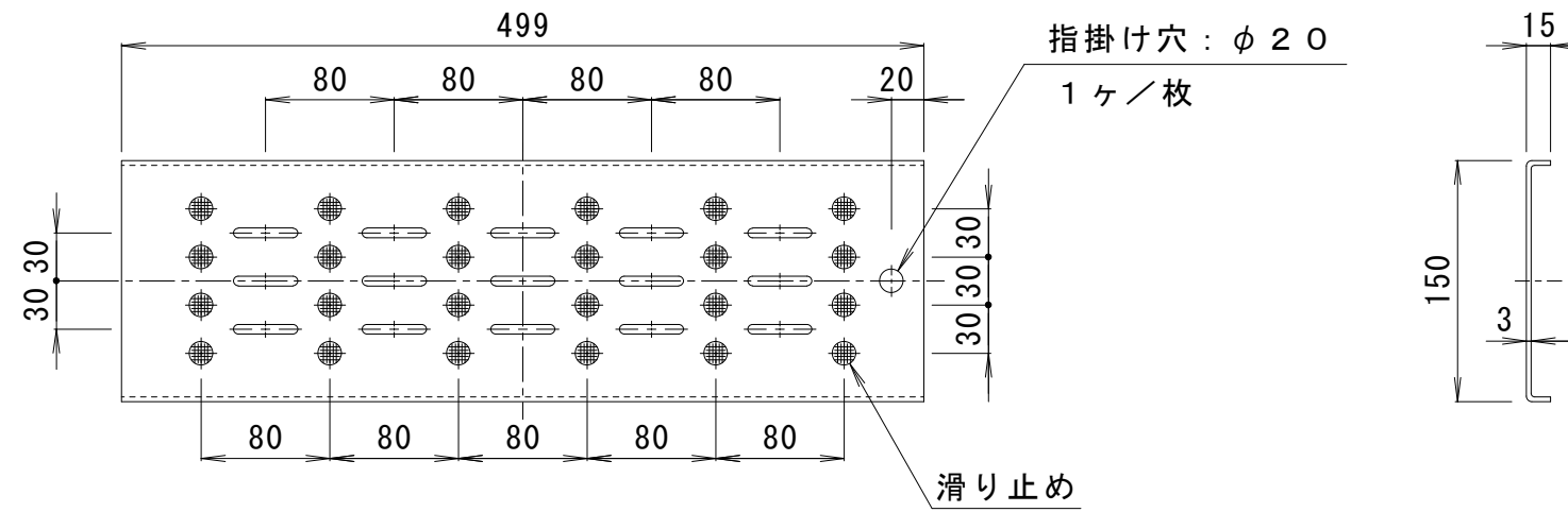
詳細図 S = 1 : 5
