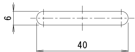
排水穴詳細図 S = 1 : 1
