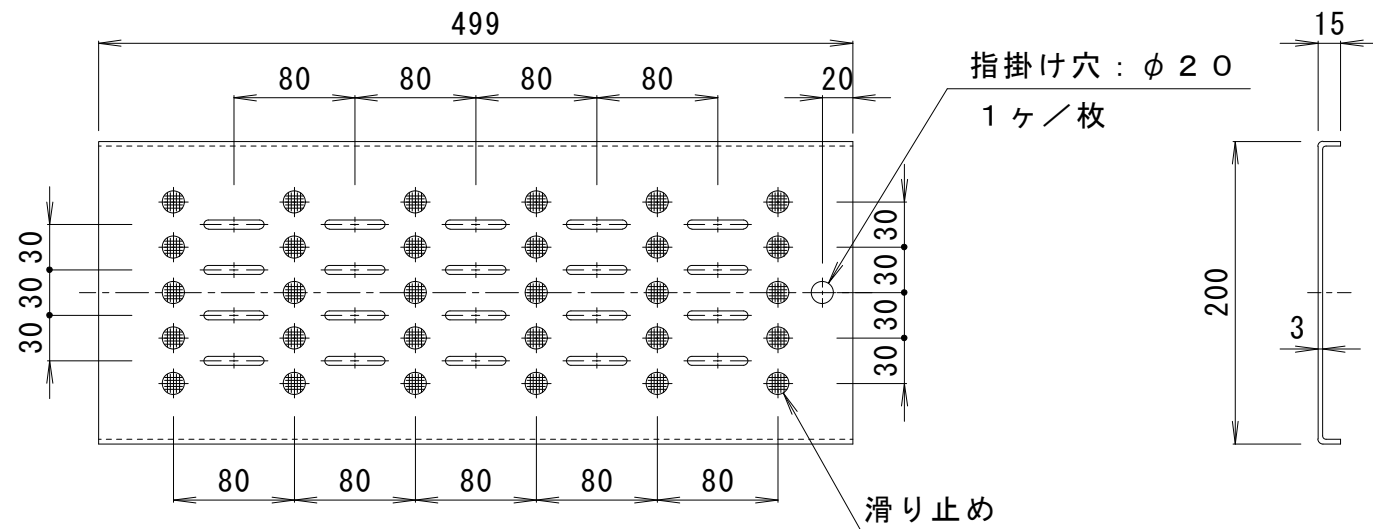
詳細図 S = 1 : 5
