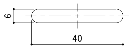
排水穴詳細図 S = 1 : 1
