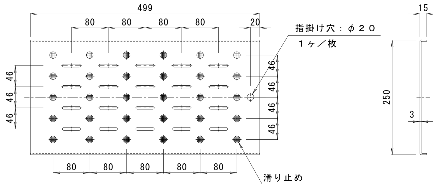
詳細図 S = 1 : 5
