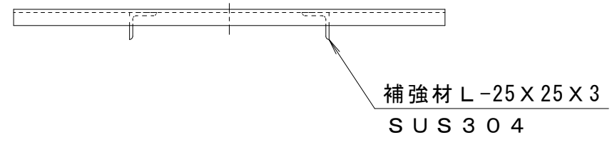
詳細図 S = 1 : 5
