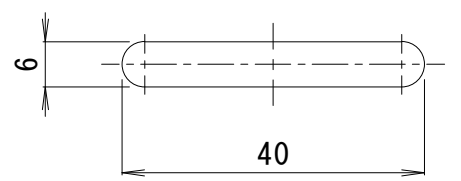
排水穴詳細図 S = 1 : 1
