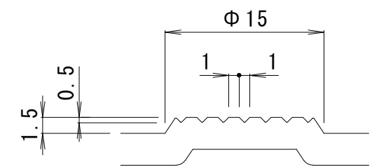
滑り止め詳細図 S = 2 : 1
