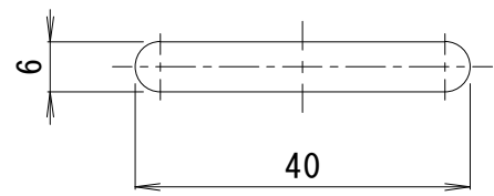
排水穴詳細図 S = 1 : 1
