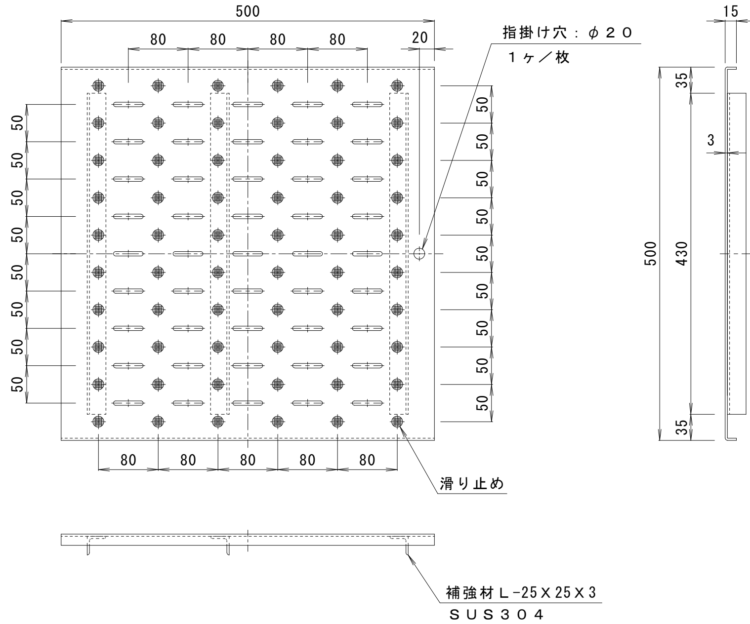
詳細図 S = 1 : 5
