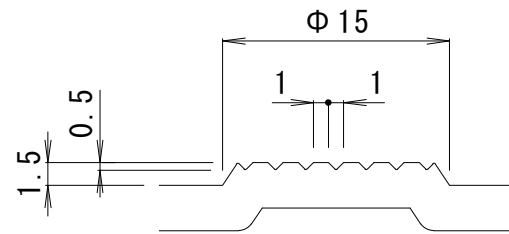
滑り止め詳細図 S = 2 : 1
