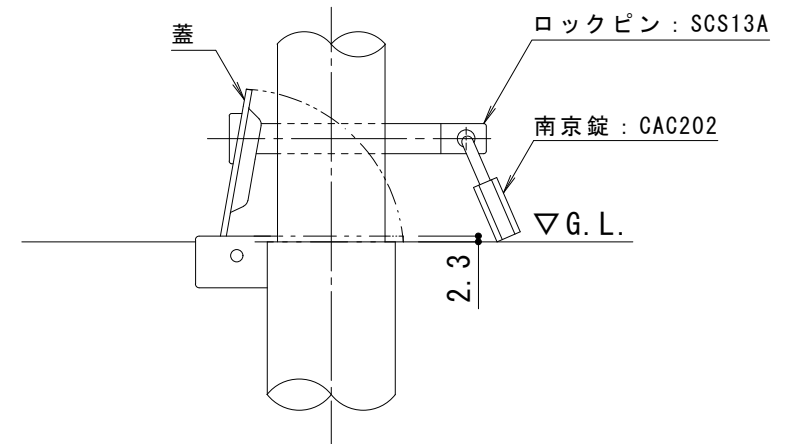
南京錠部詳細図 S = 1 : 3
