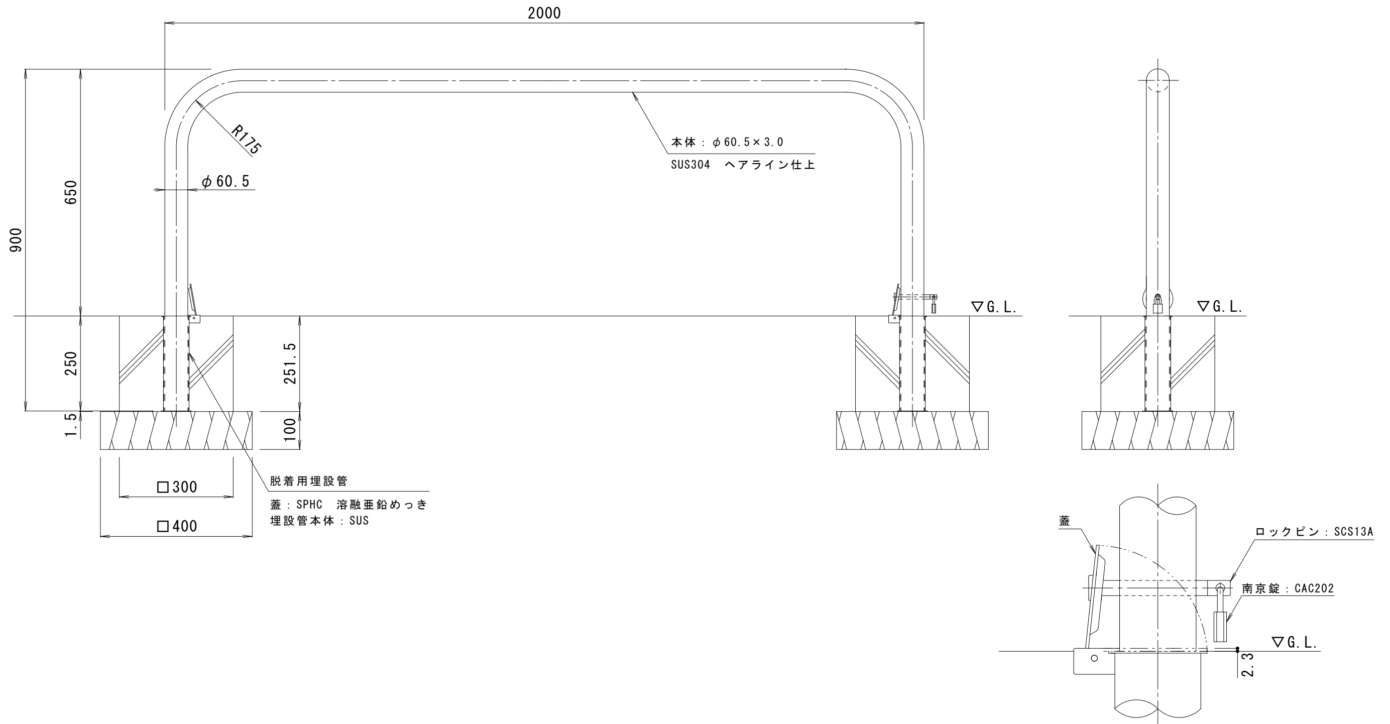
南京錠部詳細図 S = 1 : 3
