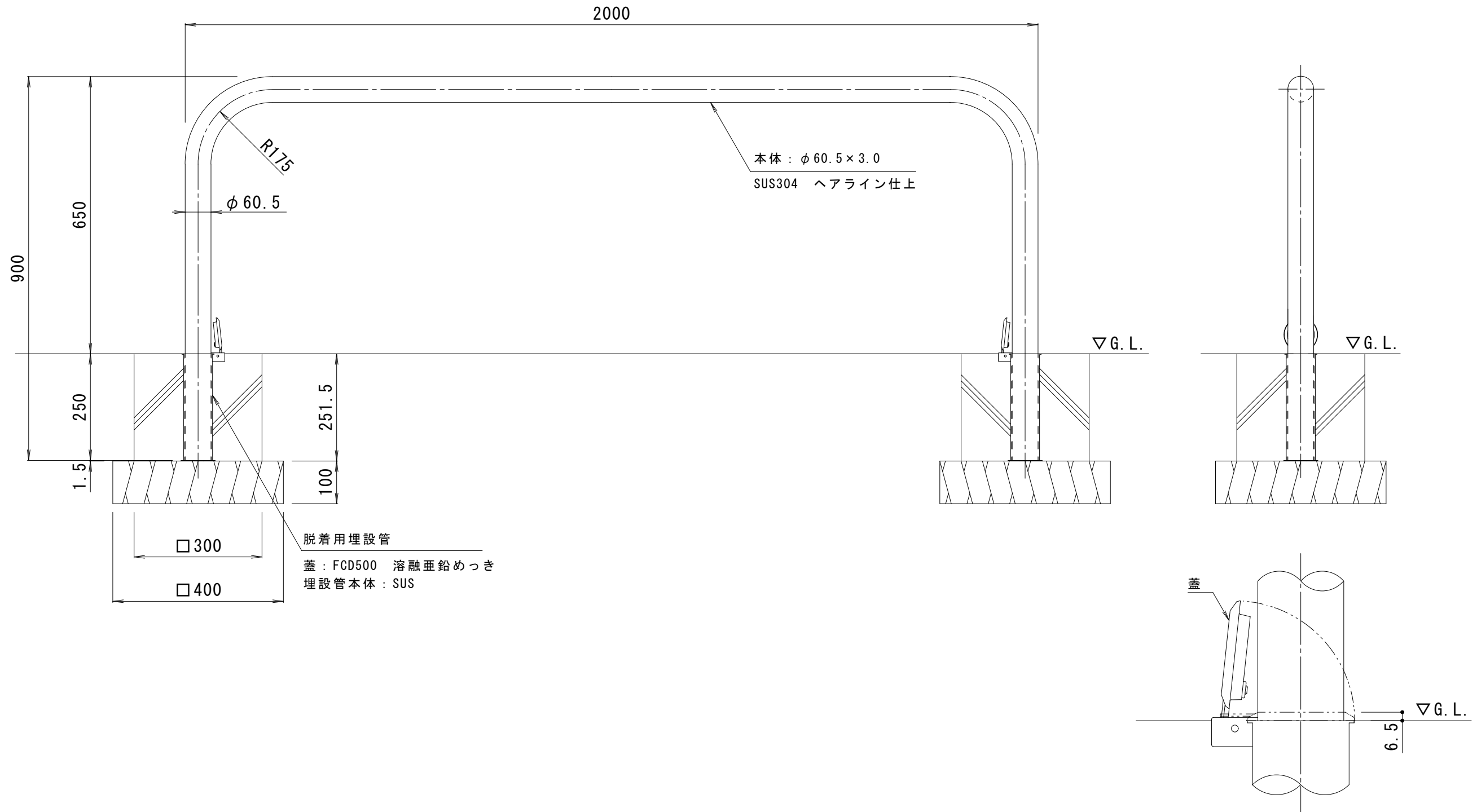
埋設管蓋部詳細図 S = 1 : 3
