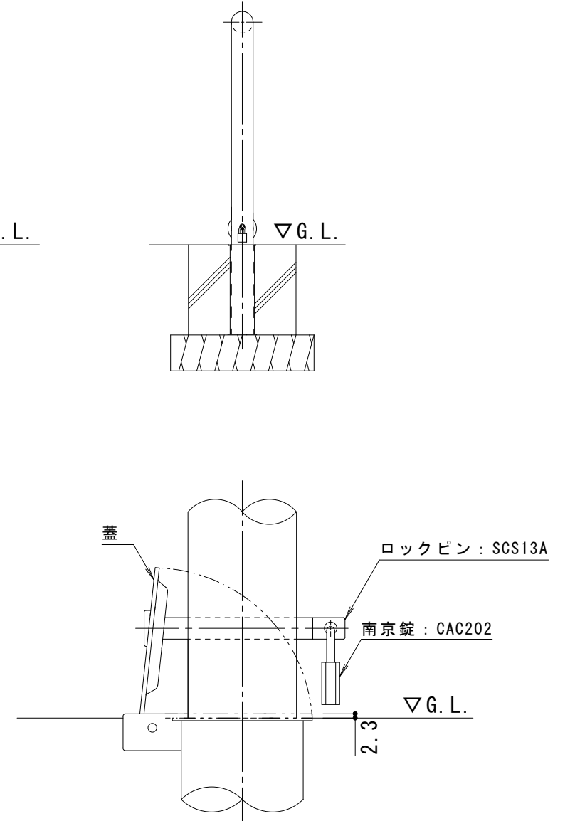
南京錠部詳細図 S = 1 : 3
