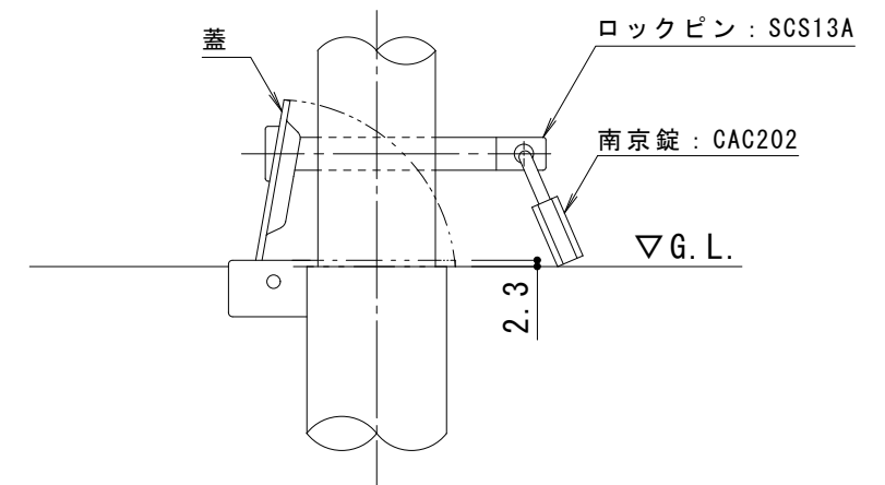
南京錠部詳細図 S = 1 : 3
