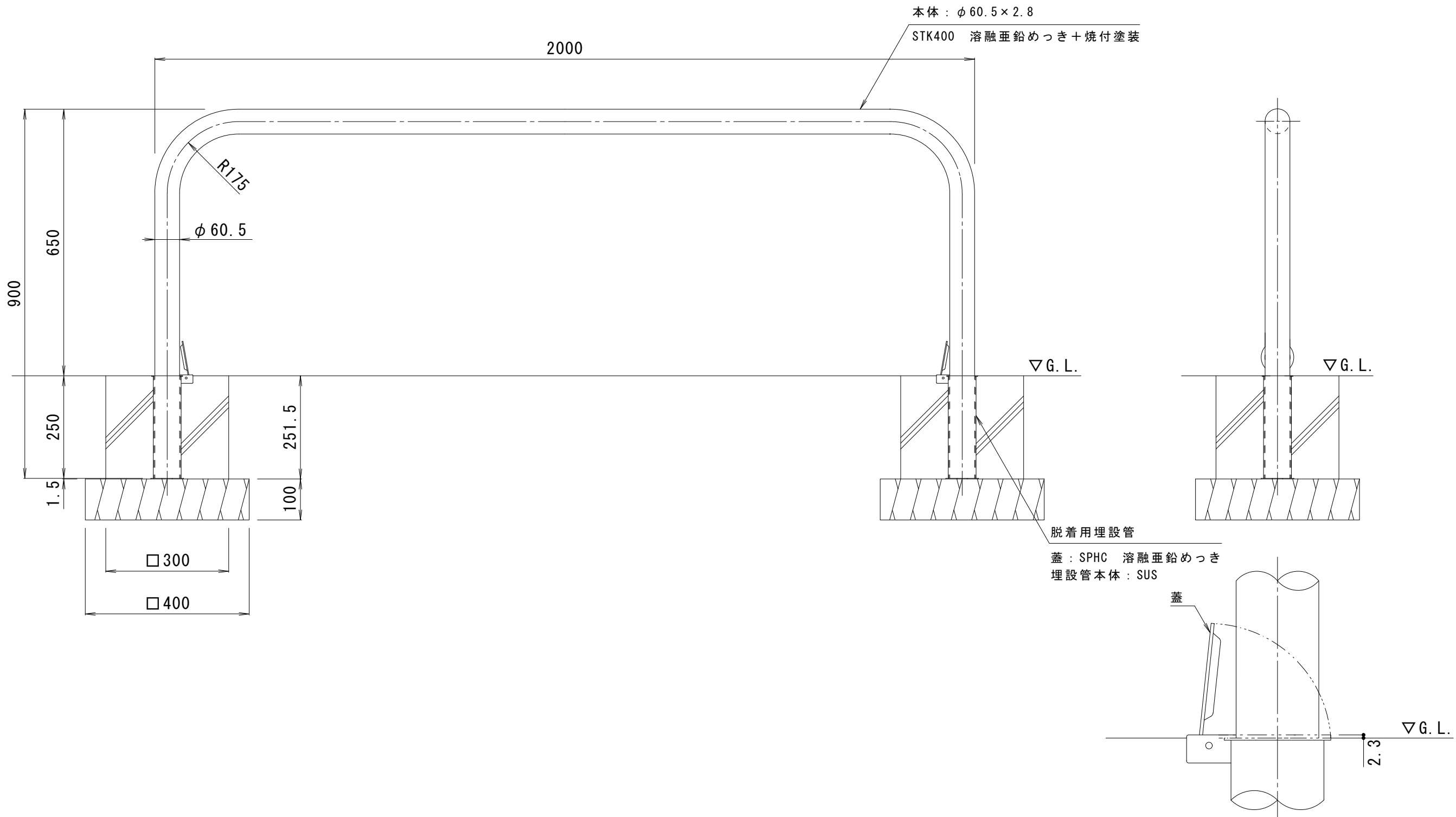
埋設管蓋部詳細図 S = 1 : 3
