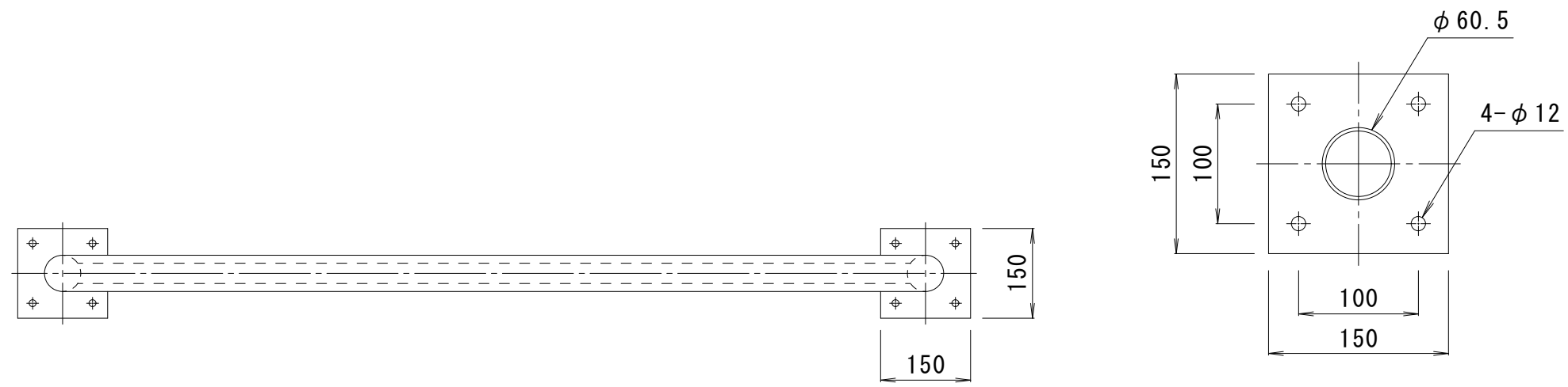
ベースプレート詳細図 S = 1 : 5
