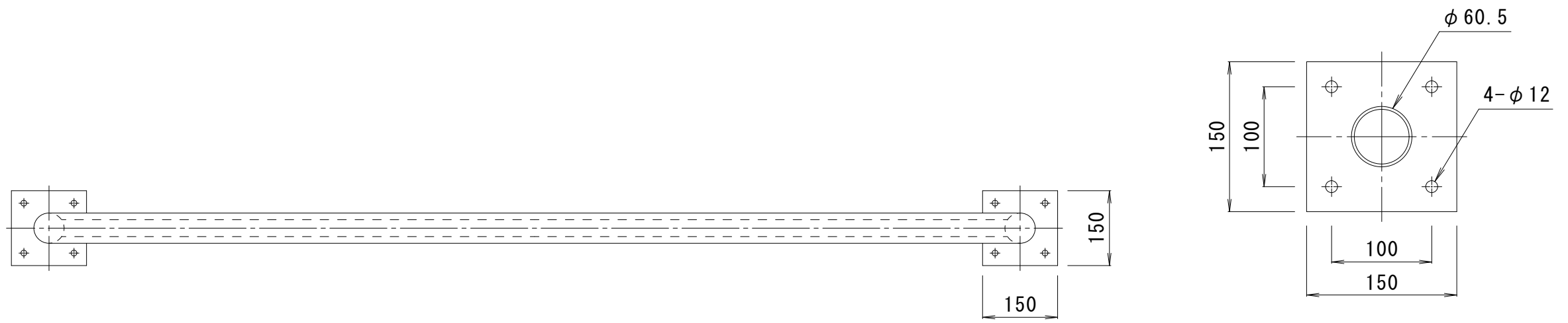
ベースプレート詳細図 S = 1 : 5
