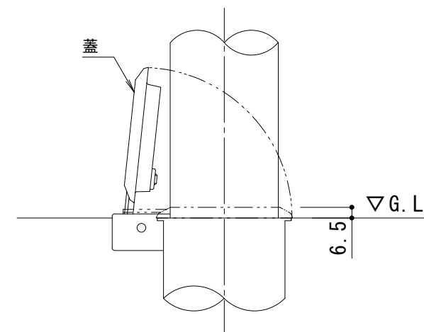
埋設管蓋部詳細図 S = 1 : 3
