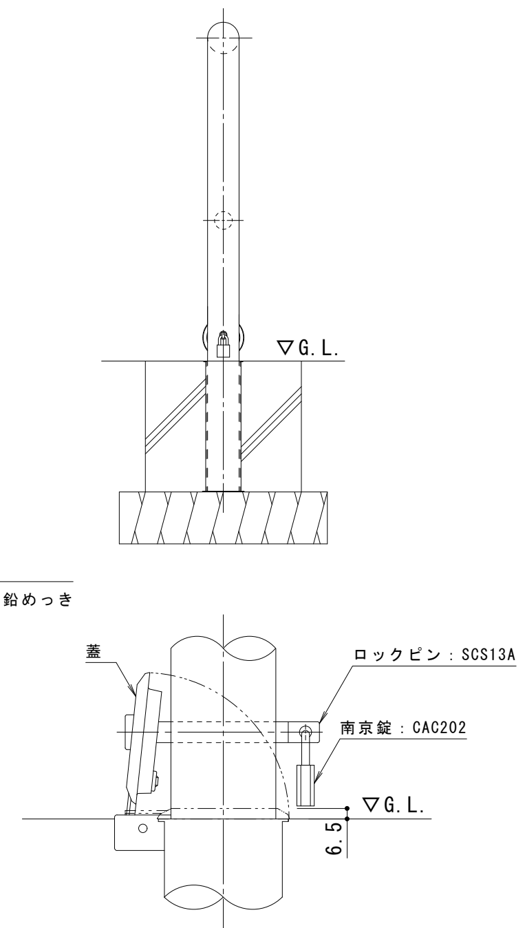
南京錠部詳細図 S = 1 : 3
