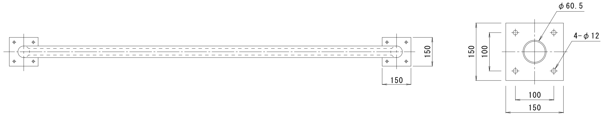
ベースプレート詳細図 S = 1 : 5
