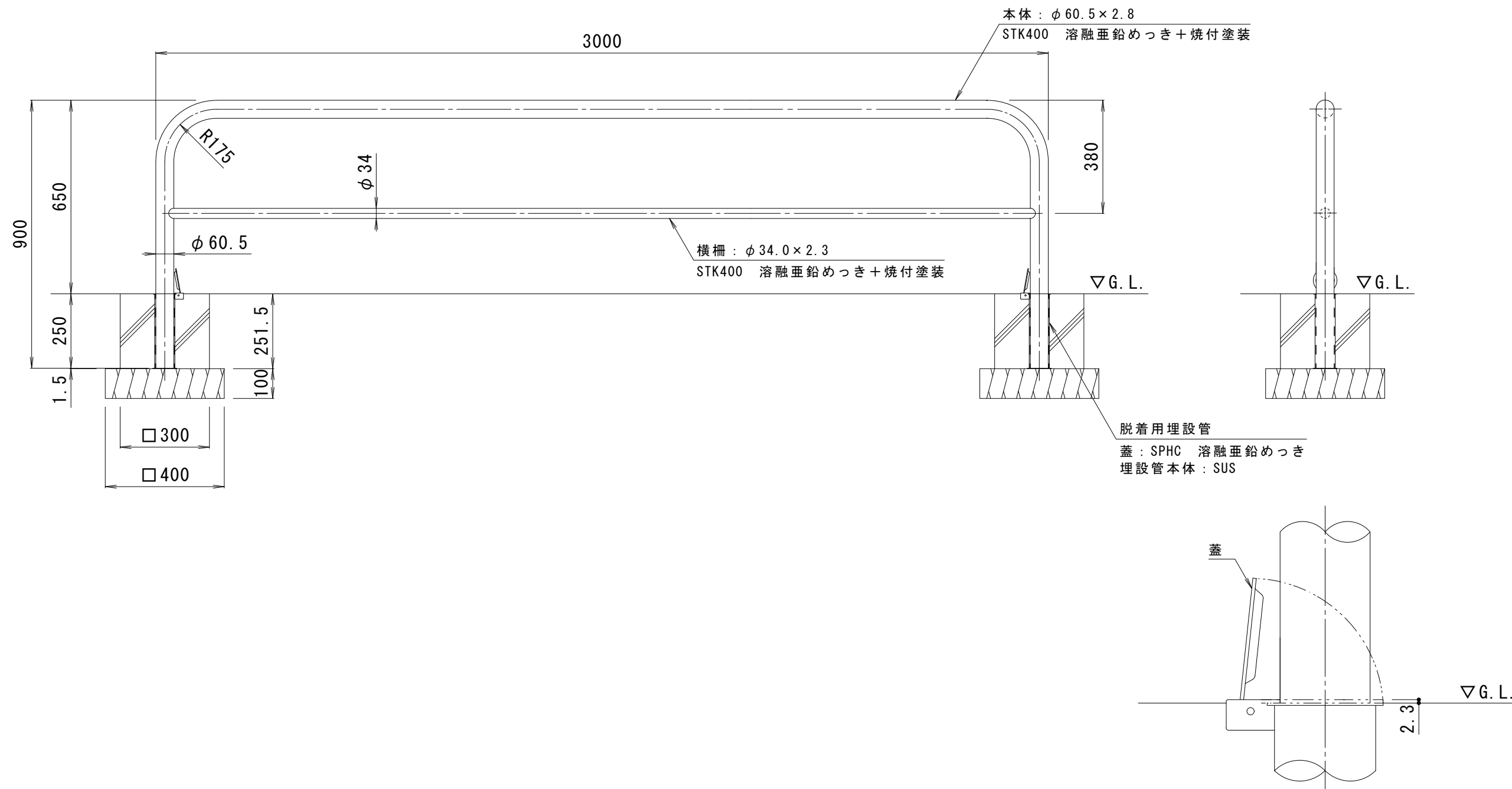
埋設管蓋部詳細図 S = 1 : 3
