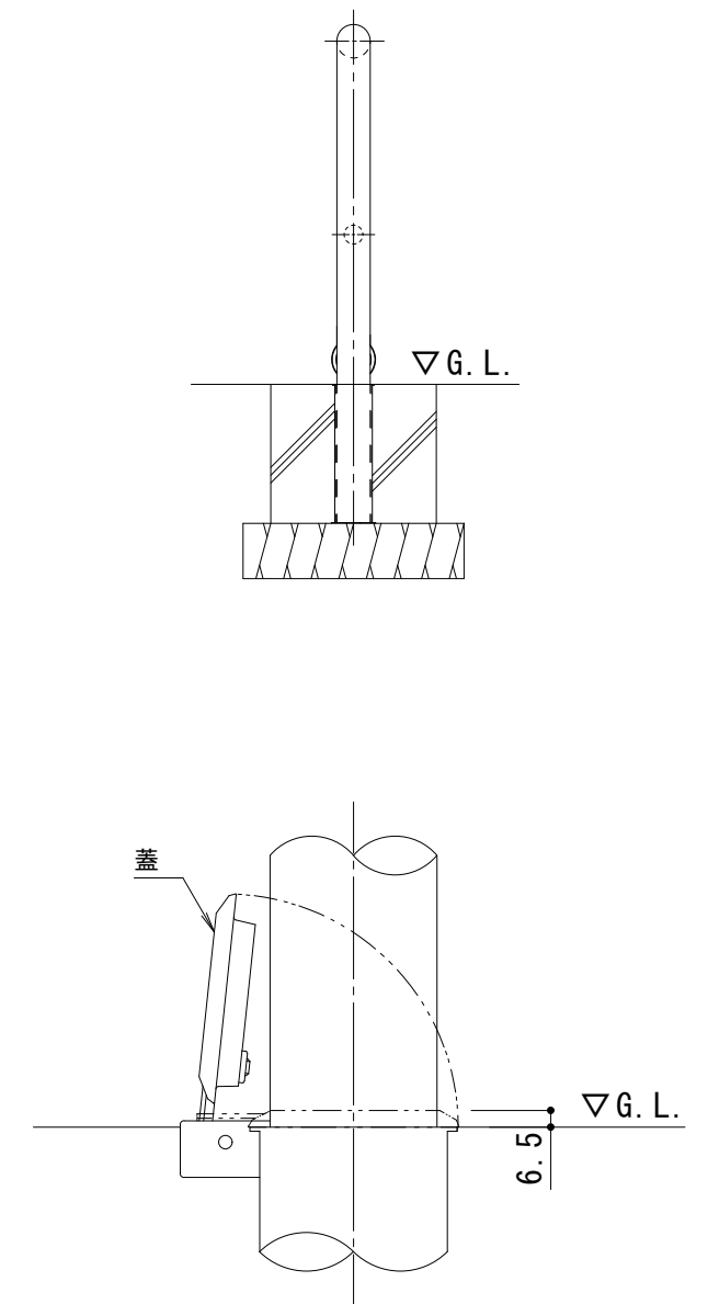
埋設管蓋部詳細図 S = 1 : 3
