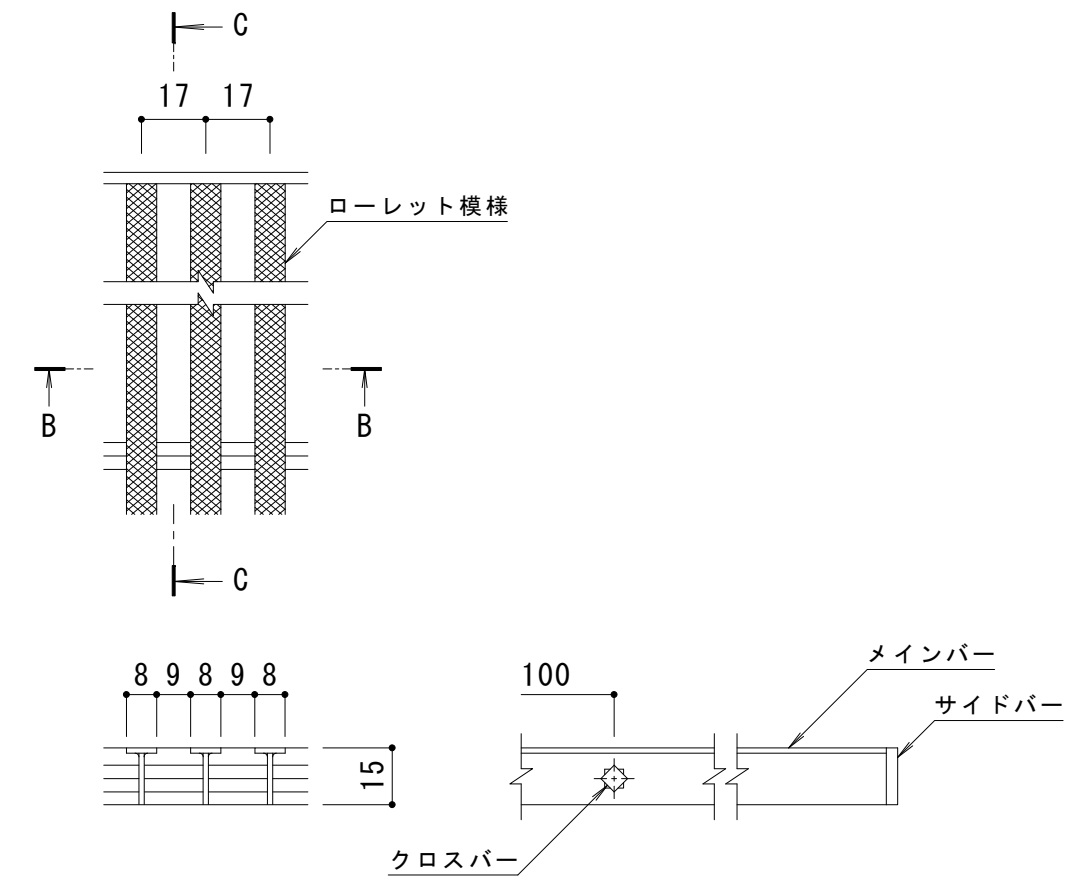
B-B断面図
