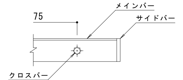
C-C断面図
