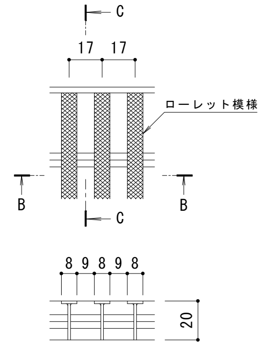
B-B断面図
