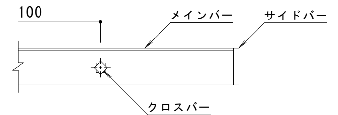
C-C断面図
