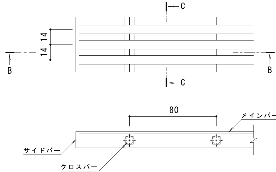
B-B断面図
