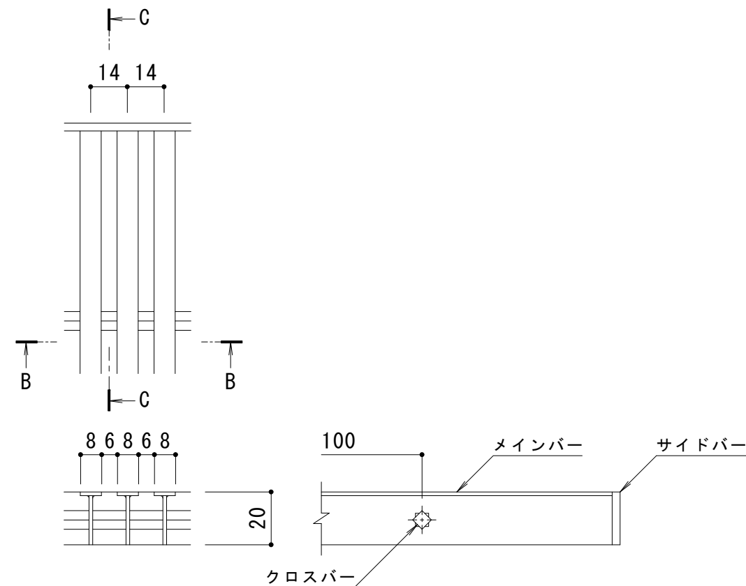
B-B断面図
