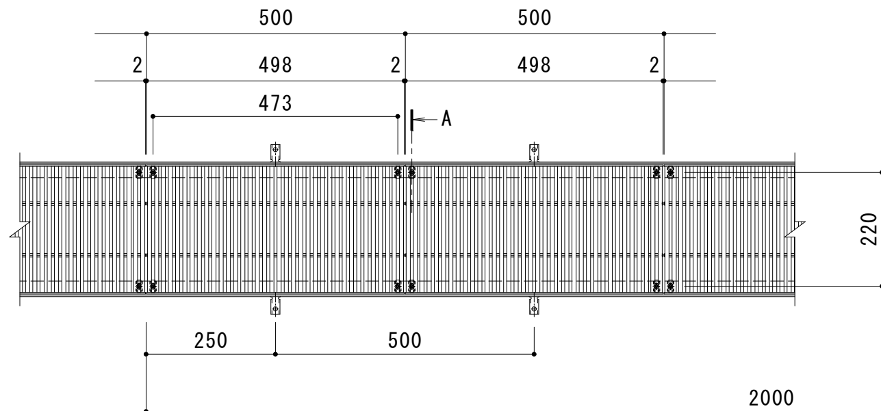
平面詳細図 S = 1 : 10
