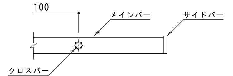
C-C断面図
