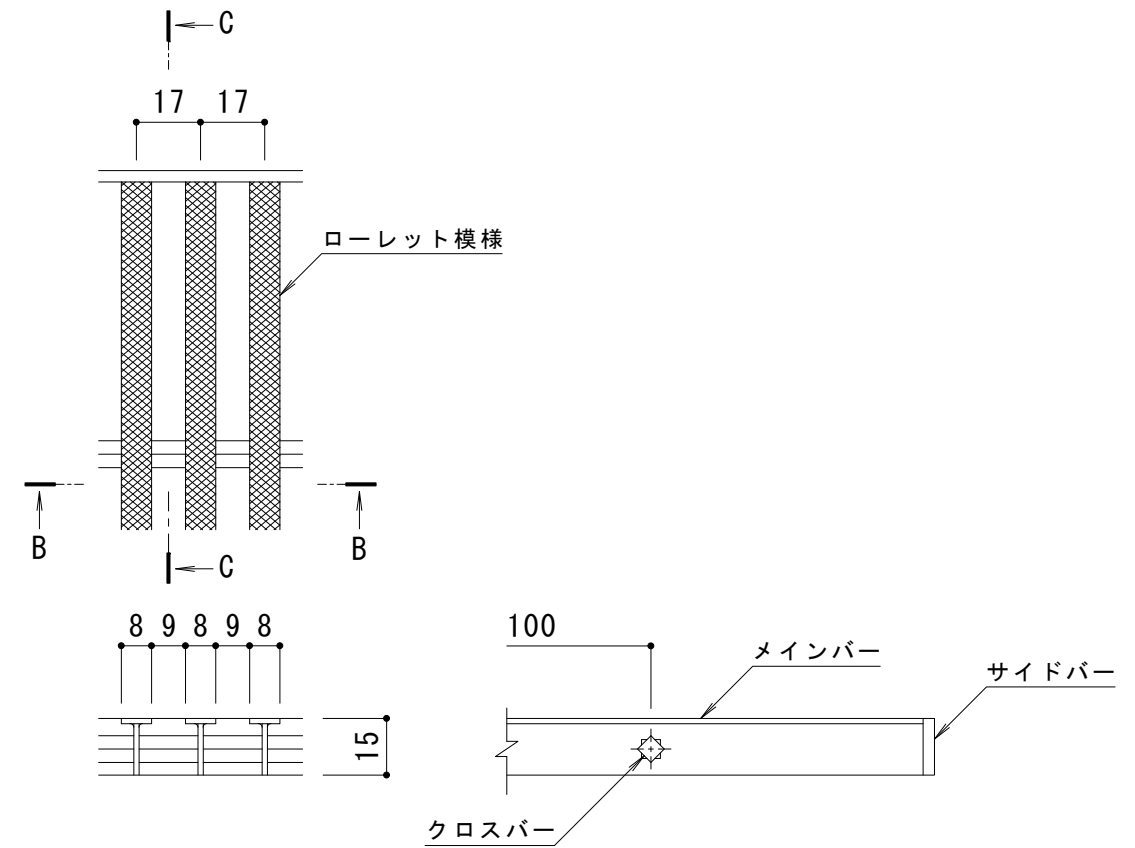
B-B断面図
