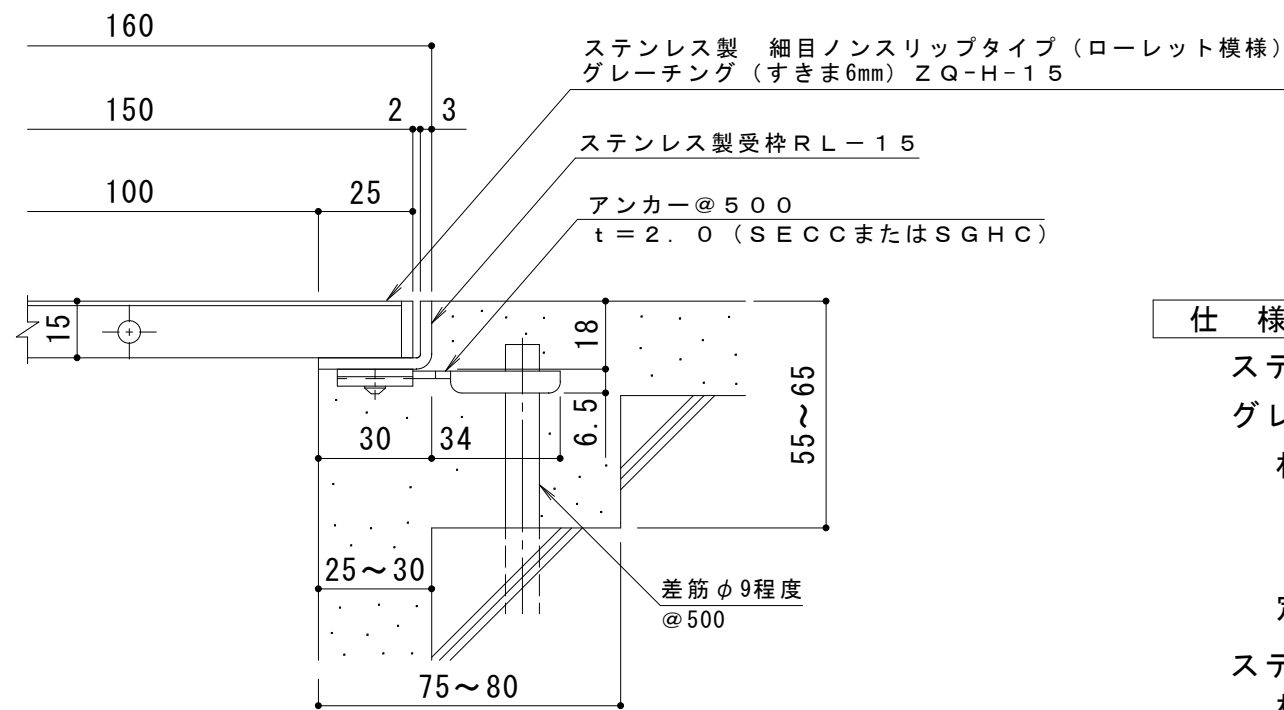
A断面詳細図 S = 1 : 2
