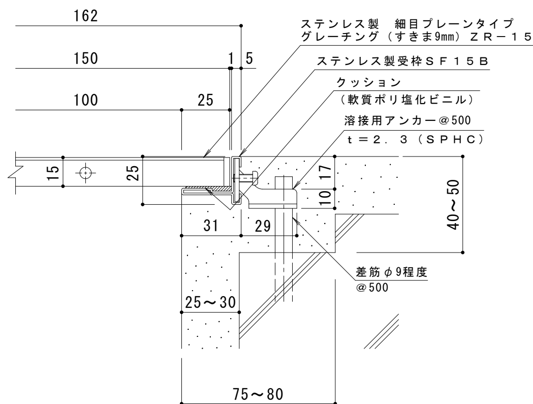
A断面詳細図 S = 1 : 2
