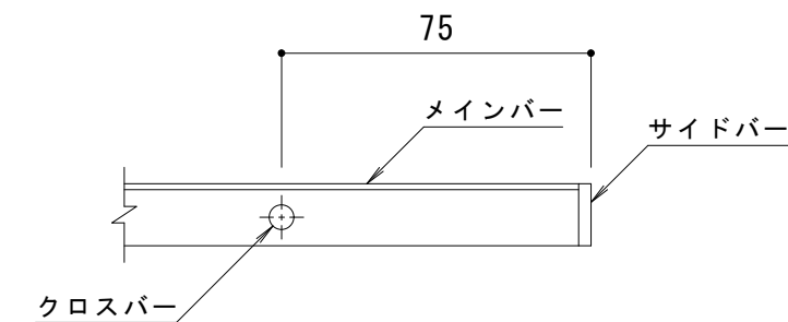
C-C断面図
