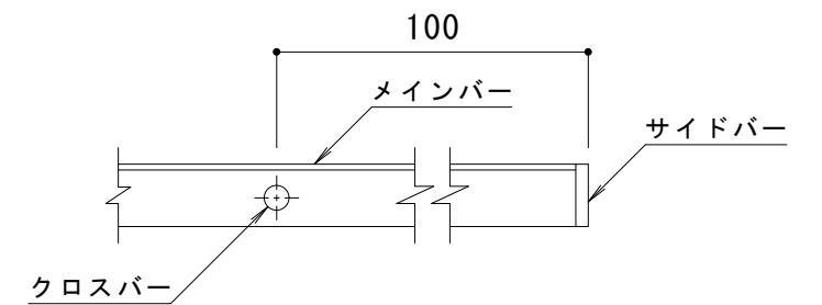
C-C断面図
